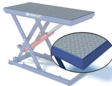
Чечевичное алюминиевое покрытие
