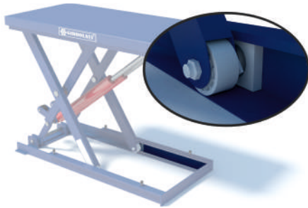
Защита от опрокидывания
